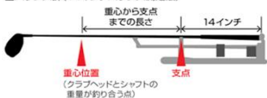
クラブバランス測定器
