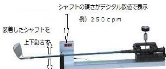
シャフト硬さを測る振動数計
